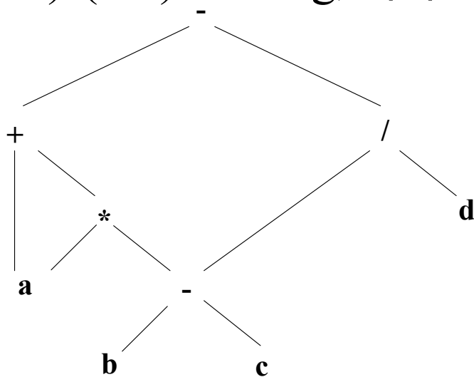
图7.5 a+a*(b-c)-(b-c)/d 的dag图
